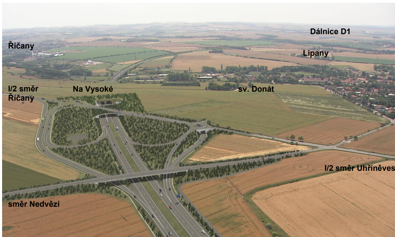
Křižovatka silničního rychlostního okruhu se silnicí I/2 (Praha – Kutná Hora), v popředí přechod silnice Kolovraty – Nedvězí po mostě přes okruh
